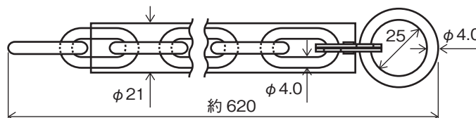
●寸法図 (mm)
