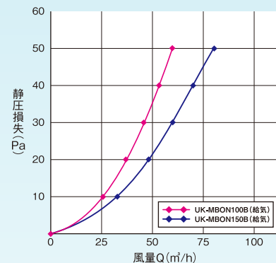
■圧損グラフ
