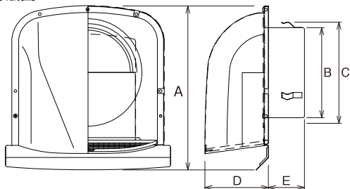
■寸法図
