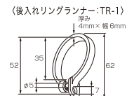
〈後入れリングランナー:TR-1〉 厚み 4mm×幅 6mm
