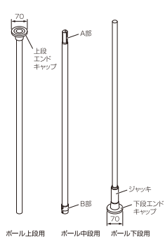
ポール上段用 ポール中段用 ポール下段用
